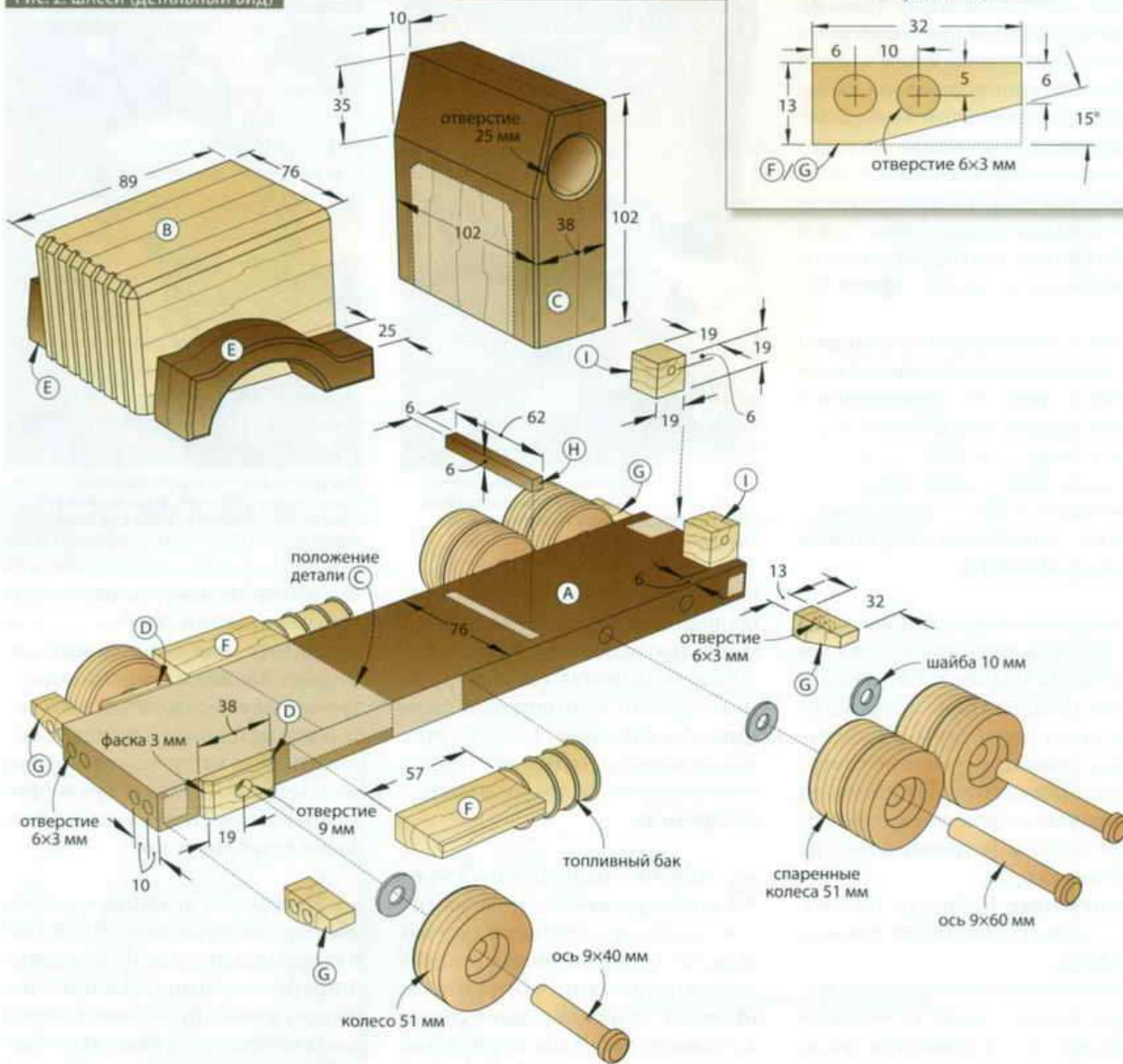
РИС. 2. ШАССИ (ДЕТАЛЬНЫЙ ВИД)
